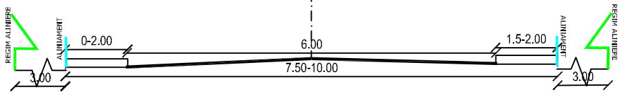
Profil strazi secundare a-a propus 1/100
